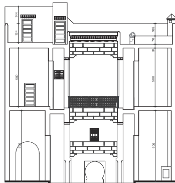
COUPE AA
